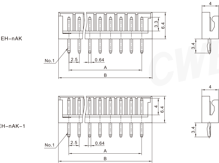
阳连接器 (立式，直插，含小弯) Header (V, DIP, W/Kink)
