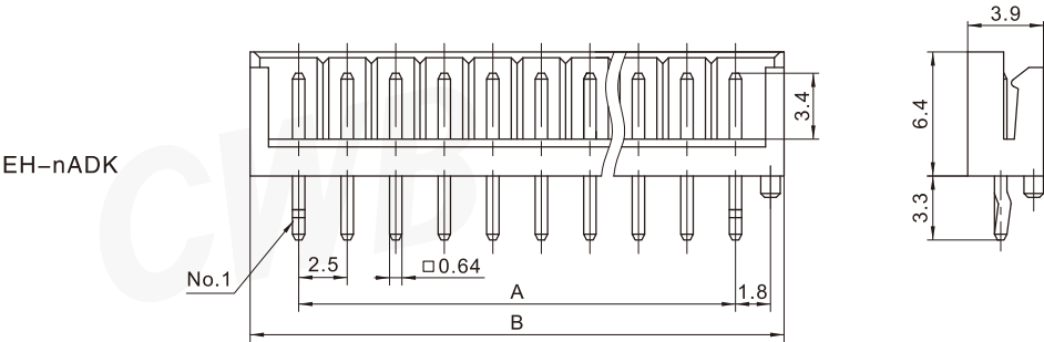
阳连接器 (立式，直插，含定位柱，含小弯) Header (V, DIP, W/Boss, W/Kink)
