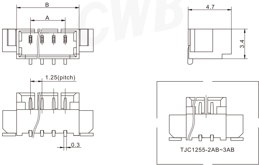
阳连接器 (卧式，表面装贴) Header (H, SMT)
