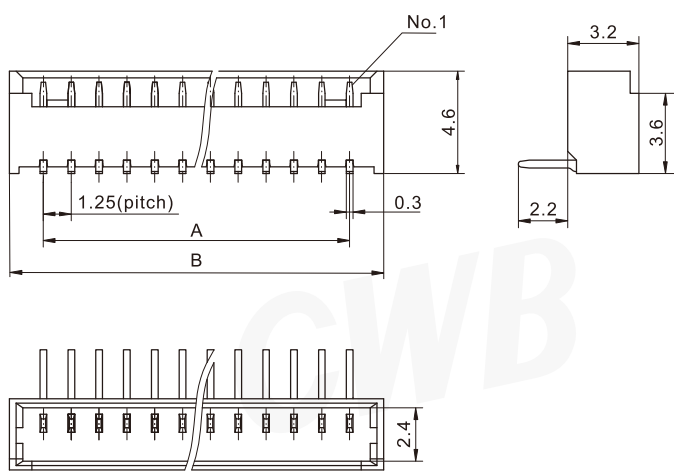
阳连接器 (卧式，直插) Header (H, DIP)
