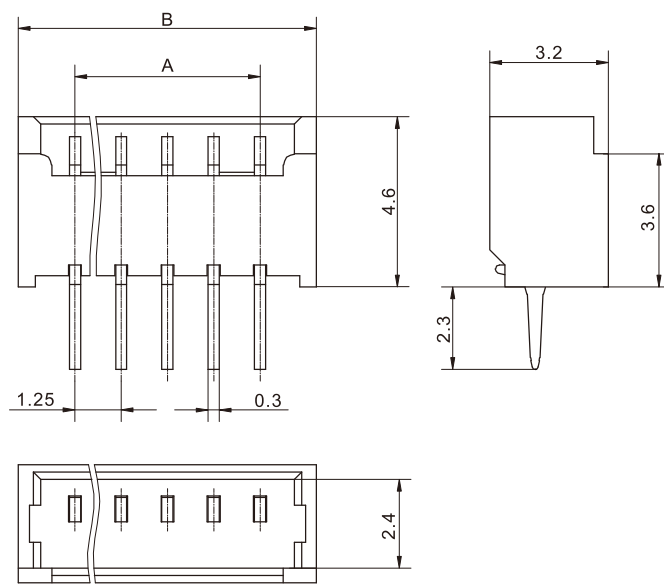
阳连接器 (立式，直插) Header (V, DIP)
