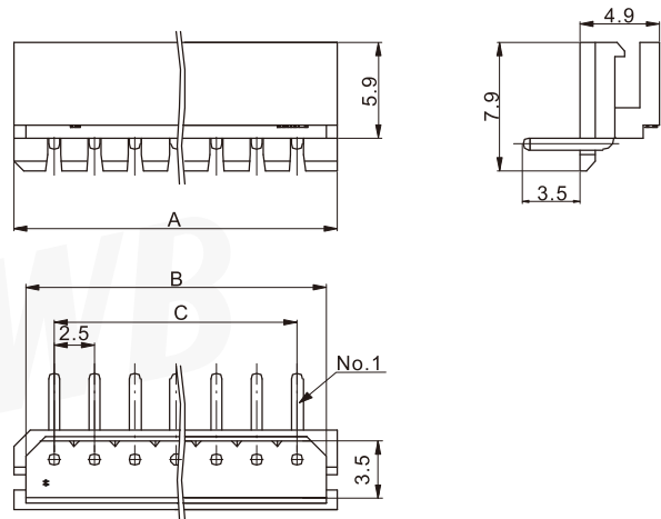
阳连接器 (卧式，直插，带挡板) Header (H, DIP, W/PCB stabilizer)
