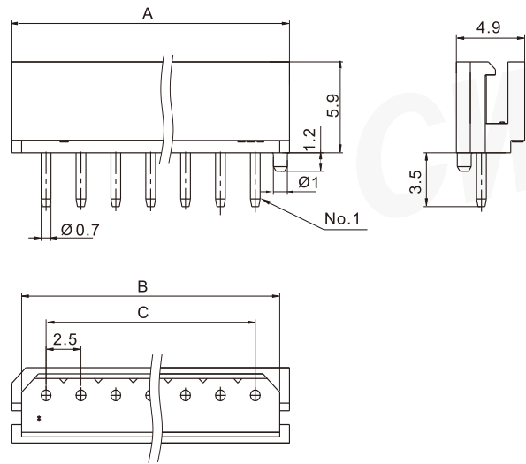
阳连接器 (卧式，直插，带挡板) Header (H, DIP, W/PCB stabilizer)
