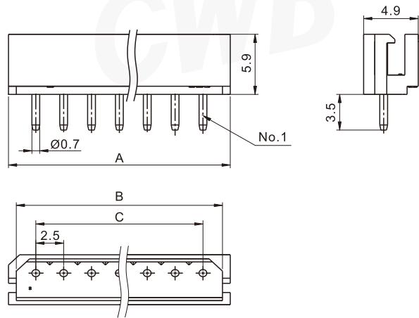
阳连接器 (立式，直插，含定位柱) Header (V, DIP, W/Boss)
