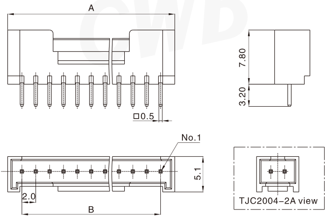
阳连接器 (立式, 直插) Header (V, DIP)
