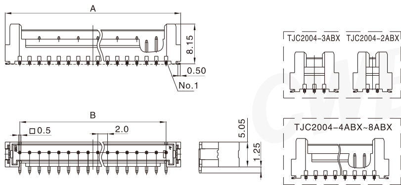
阳连接器 (立式，表面装贴，带吸嘴盖) Header (V, SMT, With cover)
