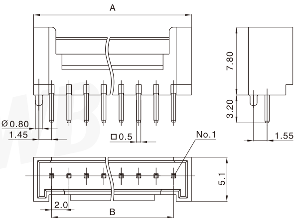
阳连接器 (立式, 直插, 带定位柱) Header (V, DIP, W/boss)
