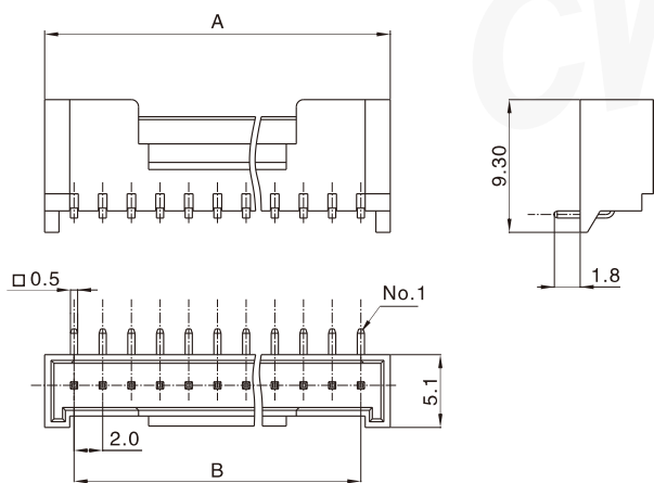
阳连接器 (卧式，直插，带挡板) Header (H, DIP, W/PCB stabilizer)
