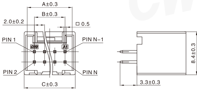
阳连接器 (立式，直插) Header (V, DIP)
