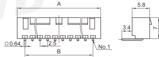
阳连接器 (弯式) WAFER (90°)
