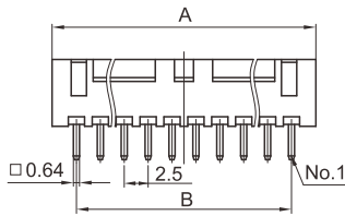
阳连接器 (弯式) HEADER (90°)
