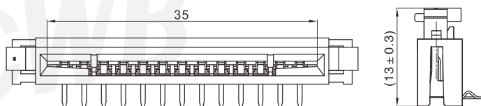
锁紧片安装示意图
