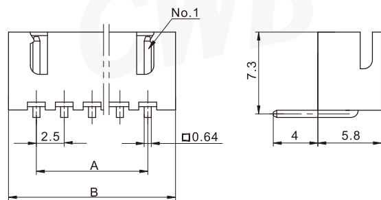
阳连接器 (立式，直插，含定位柱，含小弯) Header (V, DIP, W/Boss, W/Kink)
