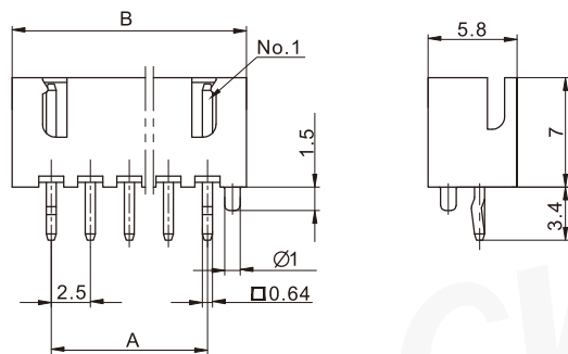
阳连接器 (卧式，直插，带挡板，含小弯) Header (H, DIP, W/PCB stabilizer, W/Kink)
