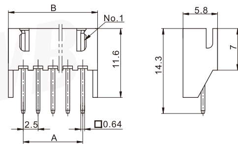
阳连接器 (立式，直插，带挡板) Header (V, DIP, W/PCB stabilizer)
