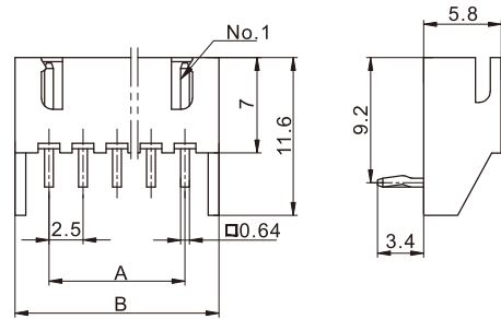
阳连接器 (立式，直插，带挡板) Header (V, DIP, W/PCB stabilizer)
