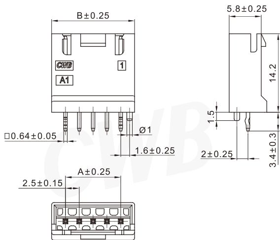
阳连接器 (立式,直插,含小弯,含定位柱 ) Header (V,DIP, W/Kink, W/Boss )
