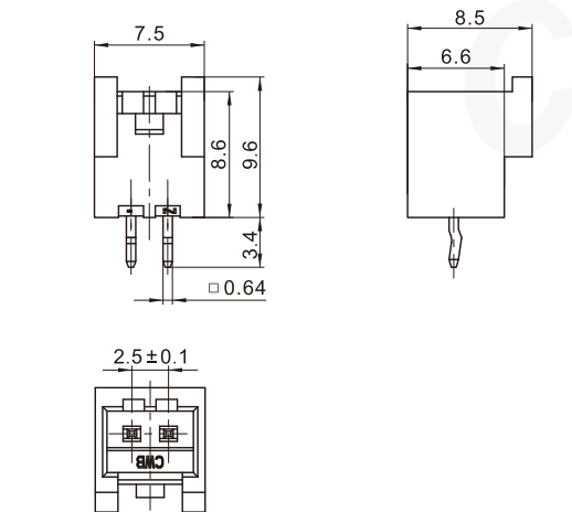
阳连接器 (立式，直插，含定位柱，含小弯) Header (V, DIP, W/Boss, W/Kink)
