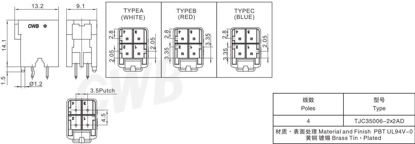
阳连接器 HEADER
