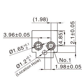
VH-2AD PCB Layout
