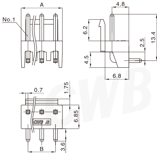
阳连接器 (卧式、直插、含挡板) Header (H、DIP、W/PCB stabilizer)
