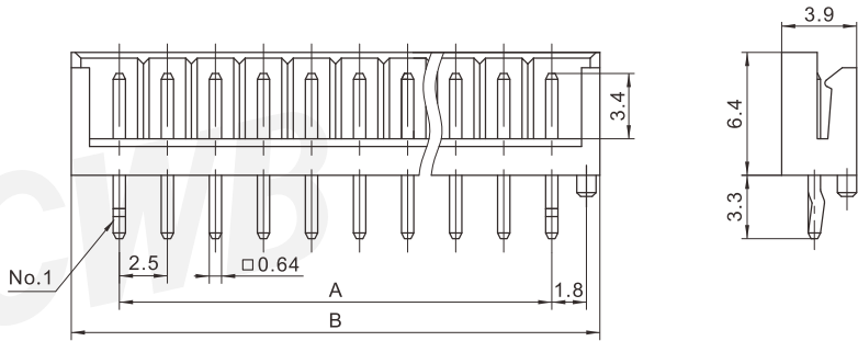
阳连接器（直式定位柱）HEADER（180°）
