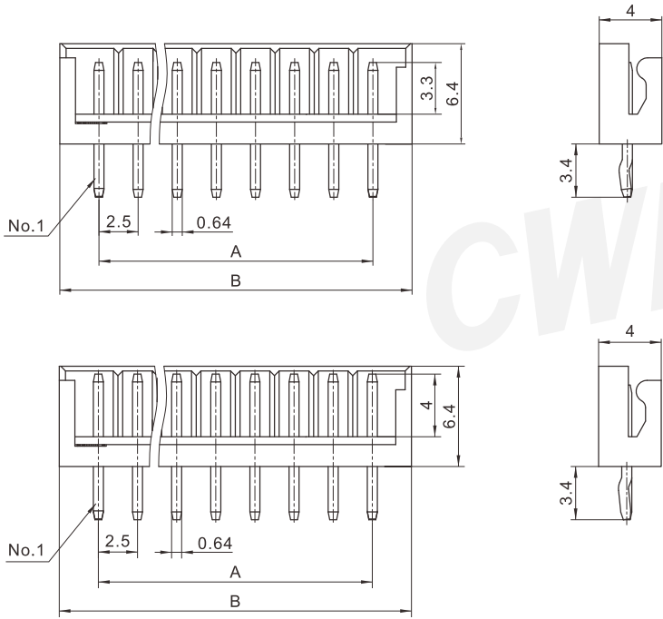
阳连接器（直式定位柱）HEADER（180°）
